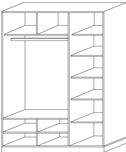
Šatník 1500 - příklad použití polic 500 a zásuvkových modulů T.
